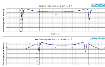
Déformation du champ magnétique avec des pertes magnétiques avec des pertes métalliques modérées
